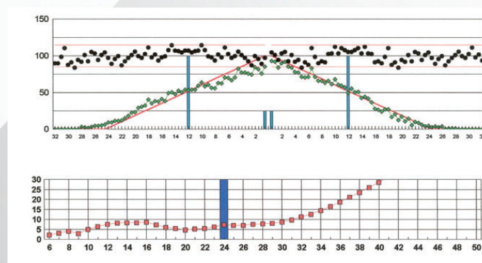
Ширина захвата: 24м, вариационный коэффициент(VK): 6,9 %, удобрение: KAS
