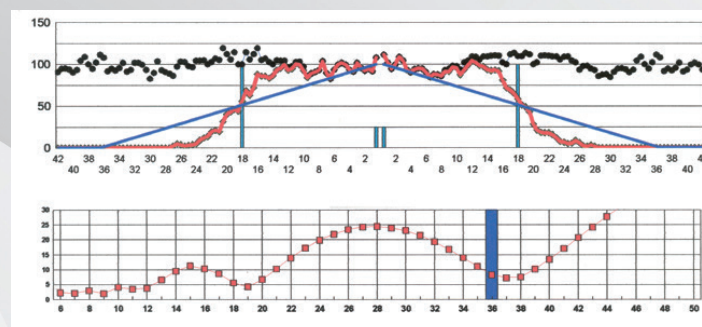
Ширина захвата: 36м, вариационный коэффициент(VK): 8,25 %, удобрение: NPK
